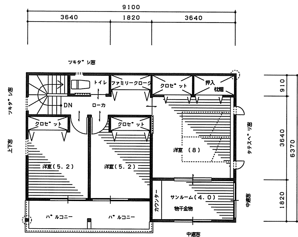
2階 平面図
