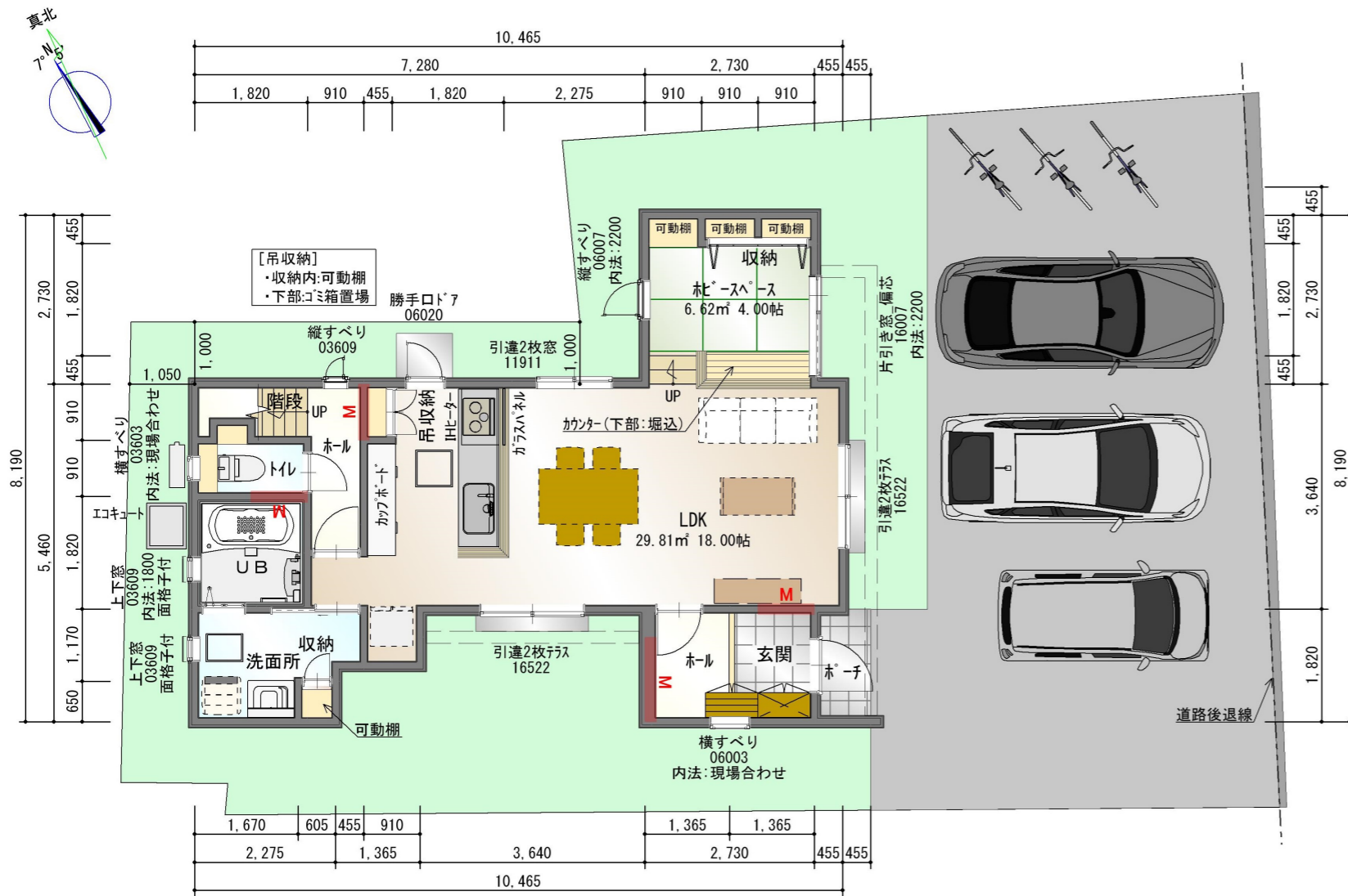
1階平面図
