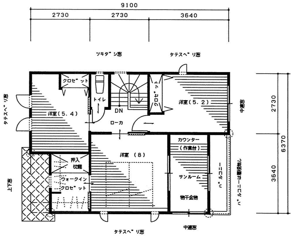
2階 平面図 1/100
