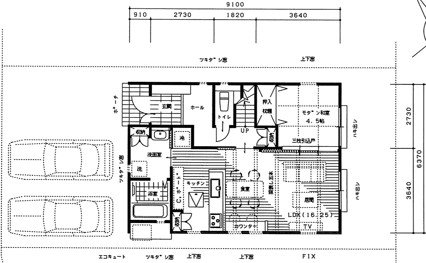
1階 平面図 1/100
