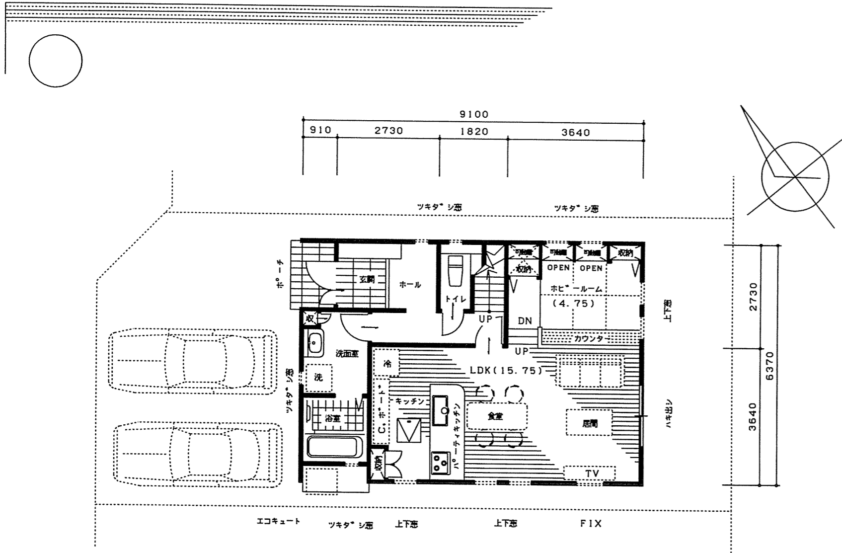
1階 平面図
