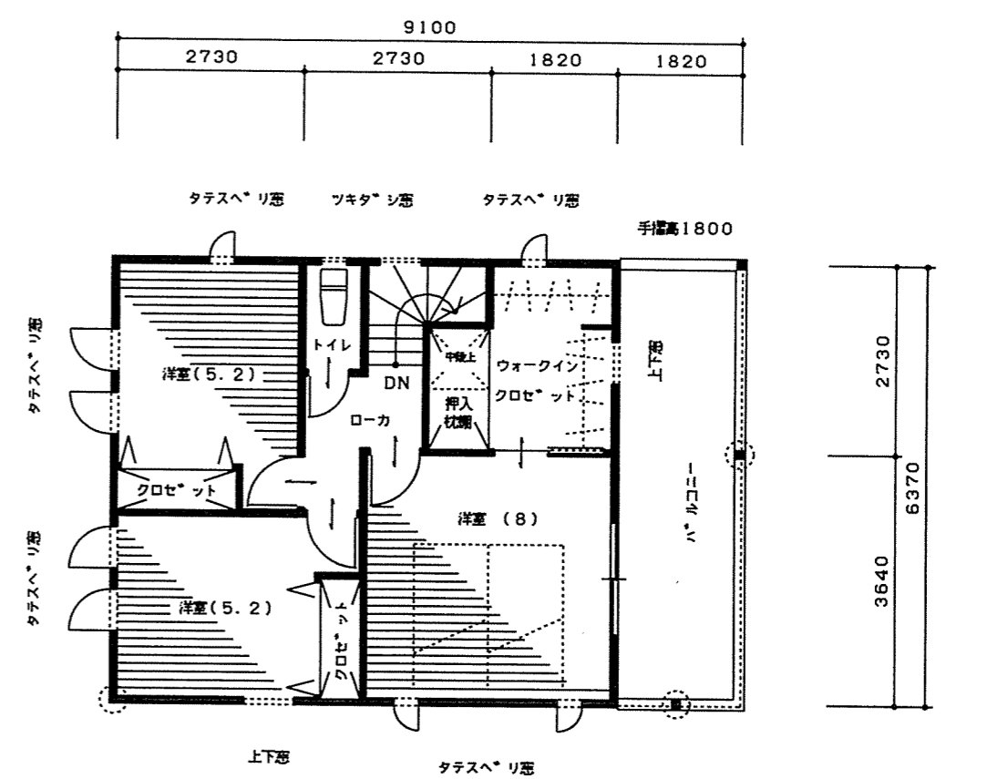
2階 平面図
