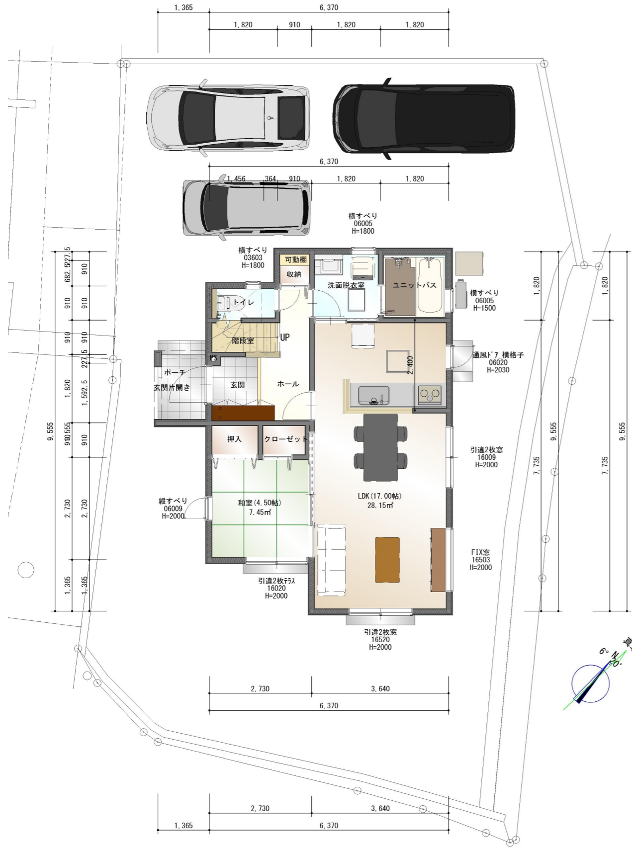
1階平面図
